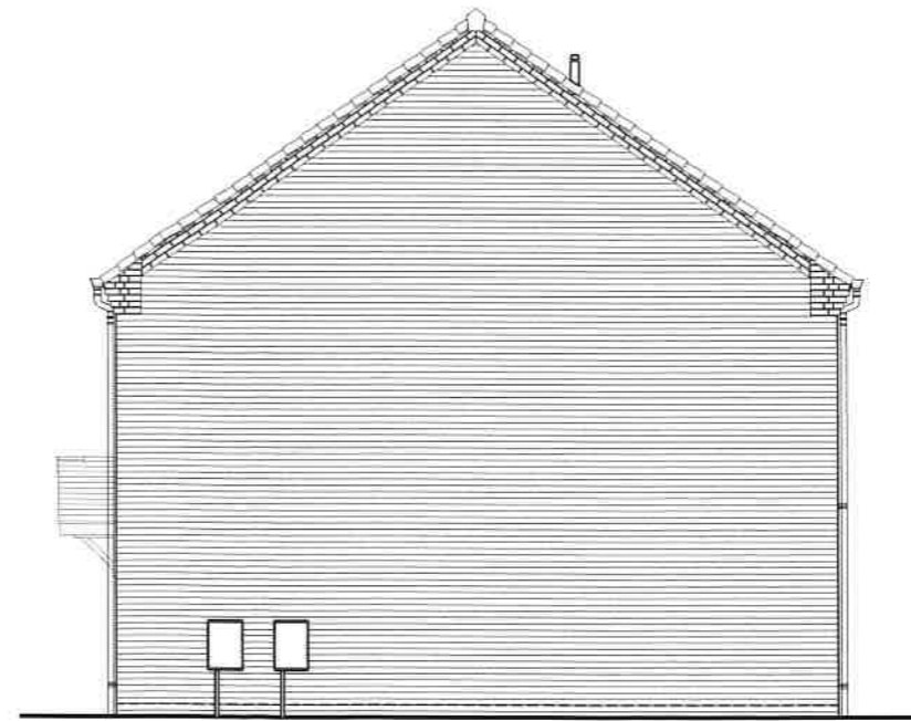
Right Elevation
